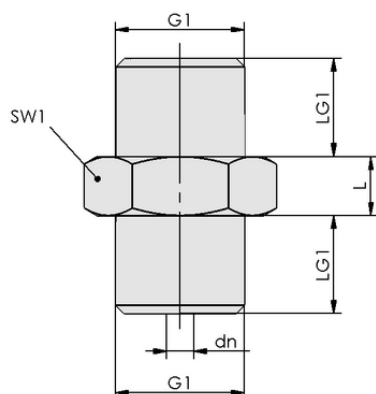
デザインデータ SW 120 G1/4-AG
