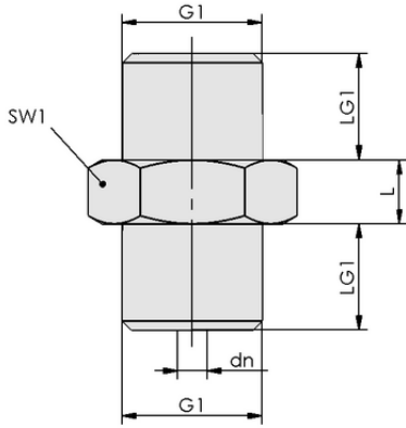
Tasarım verileri SW 70 G1/4-AG
