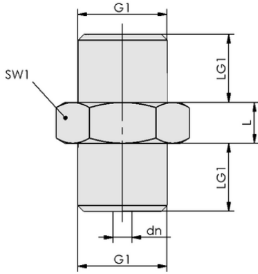
Tasarım verileri SW 70 G1/8-AG
