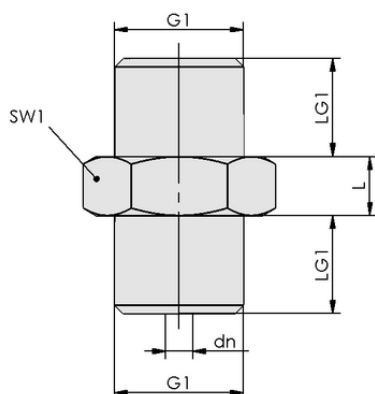
Dati di costruzione SW 50 G1/8-AG
