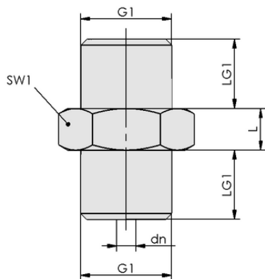
Datos de diseño SW 40 G1/8-AG
