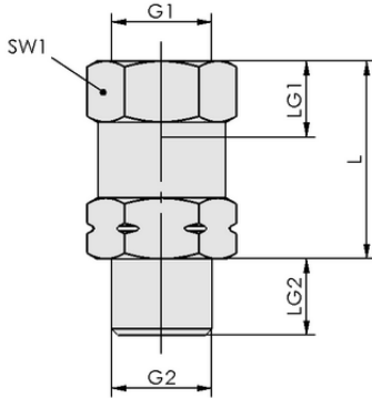
Tasarım verileri SVKG G1/8-AG
