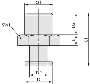
Tasarım verileri SVN G1/4-AG N014
