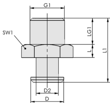
Dati di costruzione SVN G1/4-AG N014
