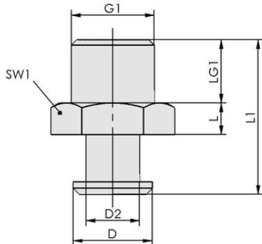
Dati di costruzione SVN G1/4-AG N011
