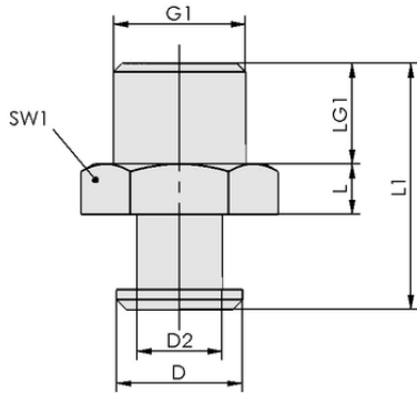
Tasarım verileri SVN G1/4-AG N019
