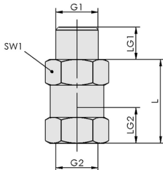
Dati di costruzione SVK G1/4-IG
