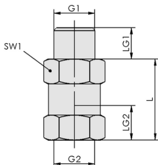
Dati di costruzione SVK G1/8-IG
