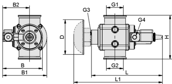
デザインデータ EMVP 50 24V-DC 3/2 NC
