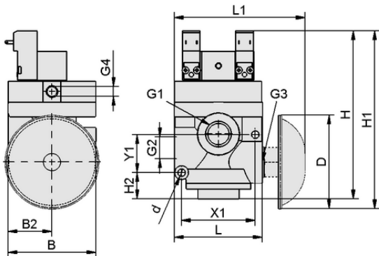
Données de construction EMVP 20 24V-DC 3/2 IMP
