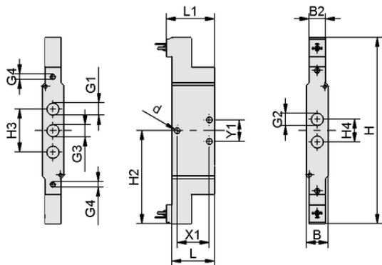
Données de construction EMVP 8 24V-DC 5/2 IMP
