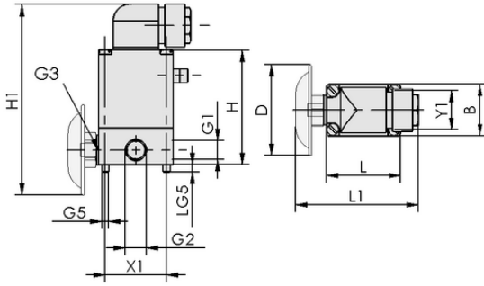
Tasarım verileri EMV 5 230V-AC 3/2 NO
