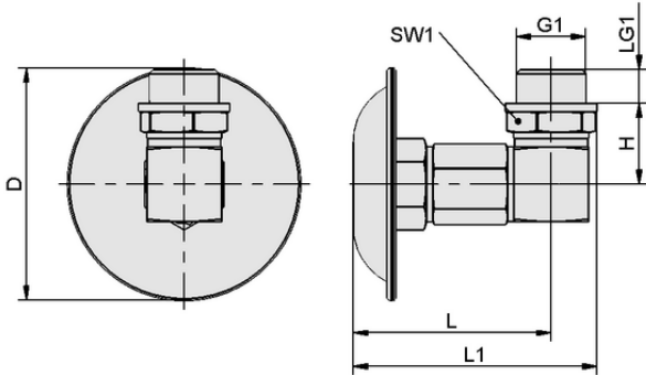
Tasarım verileri FAS 63x47 G3/8-AG EMVP-10
