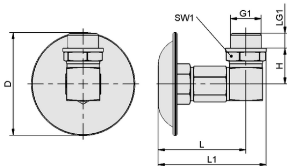
デザインデータ FAS 63x47 G3/8-AG EMVP-10
