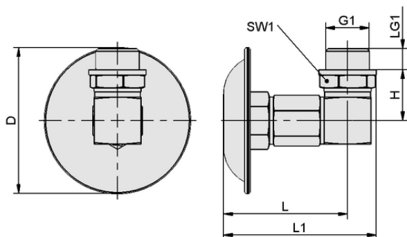
Konstruktionsdaten FAS 63x47 G3/8-AG EMVP-10
