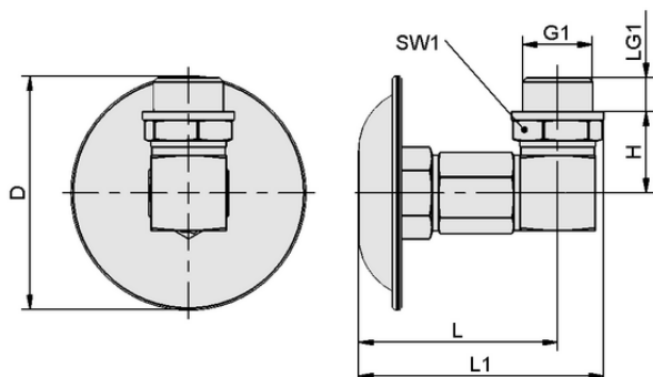
Dati di costruzione FAS 63x47 G3/8-AG EMVP-10
