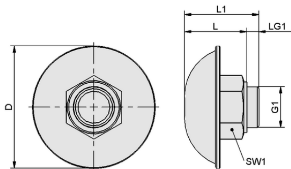
デザインデータ FAS 80x32 G1-1/4-AG EMVP-25+50
