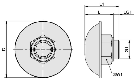
Données de construction FAS 80x32 G1-1/4-AG EMVP-25+50
