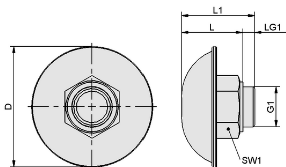
Données de construction FAS 80x38 G1-AG EMVP
