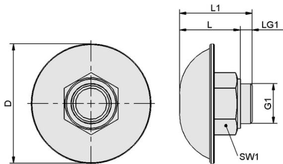
Konstruktionsdaten FAS 80x38 G1-AG EMVP
