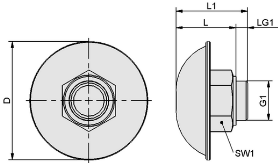
Tasarım verileri FAS 80x39 G3/4-AG
