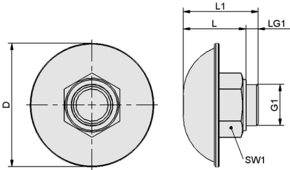
Tasarım verileri FAS 80x33.8 G1/2-AG
