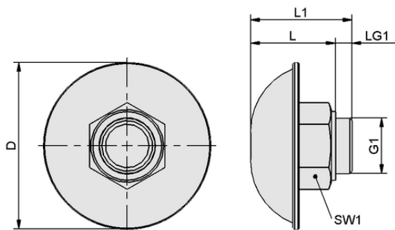
Datos de diseño FAS 63x19 G1/4-AG
