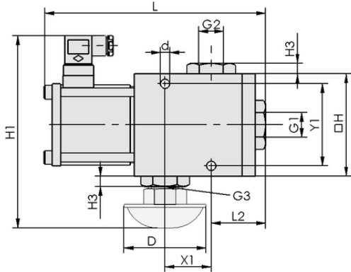
Tasarım verileri EMVO 20 230V-AC 3/2 NC
