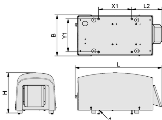
デザインデータ SBB-EVE-24V-DC-ST-VZ-LUE
