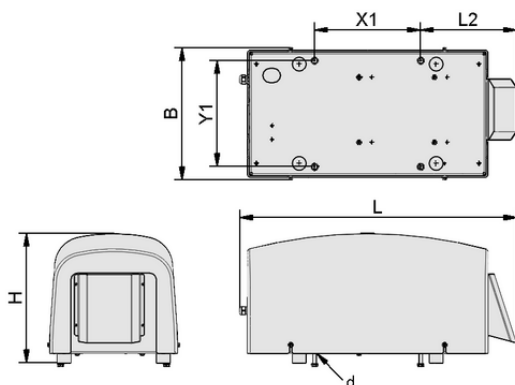
Dati di costruzione SBB-EVE-24V-DC-ST-VZ-LUE
