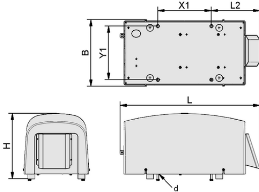
Tasarım verileri SBB-EVE-24V-DC-ST-VZ-LUE
