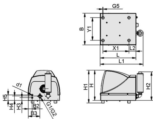
Données de construction SBB-24V-DC-ST/ABS-LUE SB
