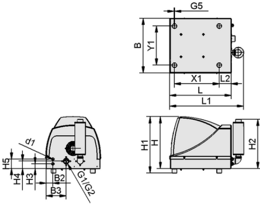
Tasarım verileri SBB-24V-DC-ST/ABS-LUE SB
