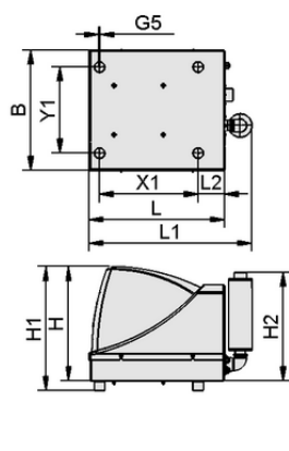
Datos de diseño SBB-24V-DC-ST/ABS-LUE SB
