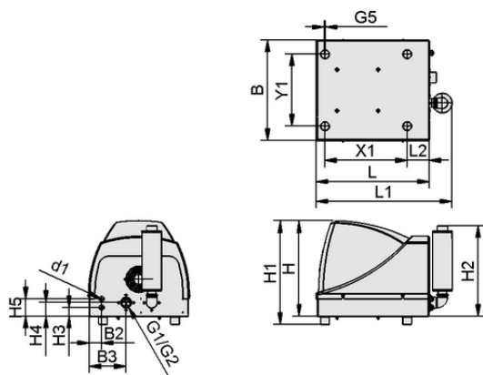
Dati di costruzione SBB-24V-DC-ST/ABS-LUE SB
