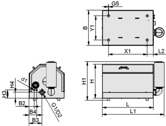
Tasarım verileri SBB-24V-DC-ST-VZ-LUE SB
