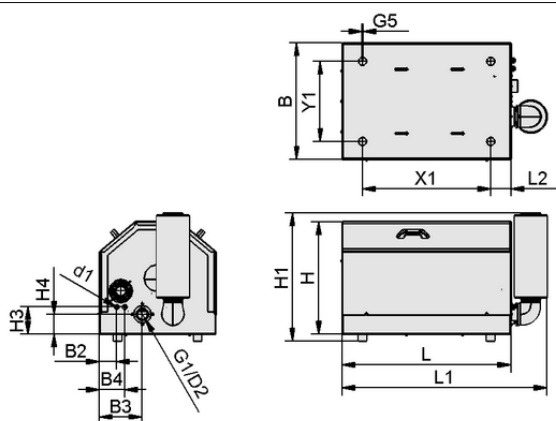
Datos de diseño SBB-24V-DC-ST-VZ-LUE SB
