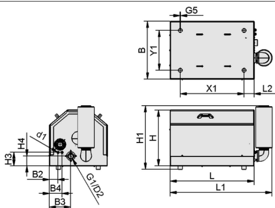
Données de construction SBB-24V-DC-ST-VZ-LUE SB
