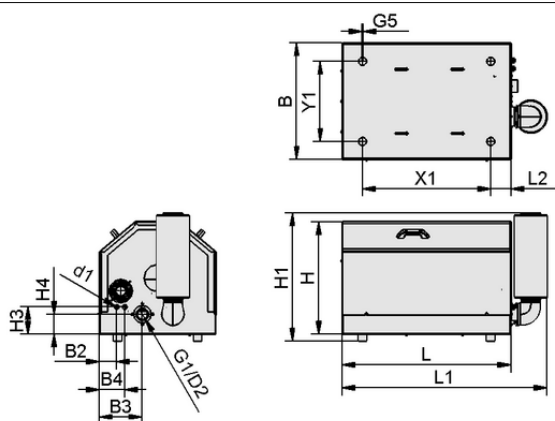
デザインデータ SBB-230V-AC-ST-VZ-LUE SB
