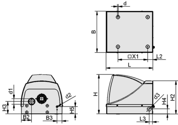
Tasarım verileri SBB-ST/ABS-VZ
