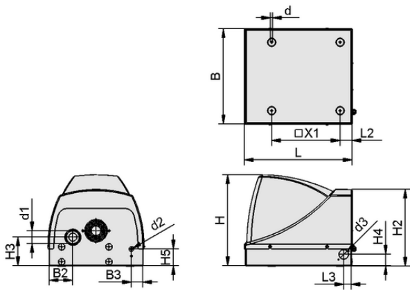
Datos de diseño SBB-ST/ABS-VZ
