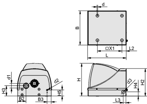
Konstruktionsdaten SBB-ST/ABS-VZ
