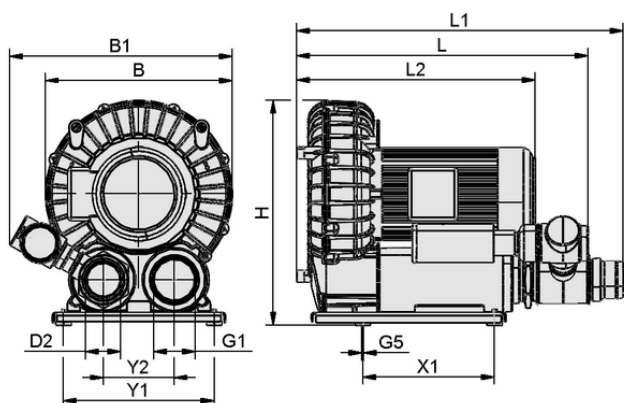
Données de construction SB 510 390 11 IE3-TYP1
