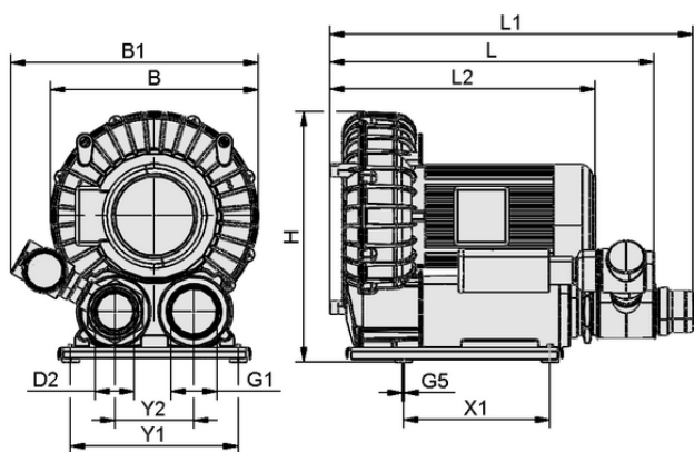
Dati di costruzione SB 435 340 6.6 IE3-TYP2
