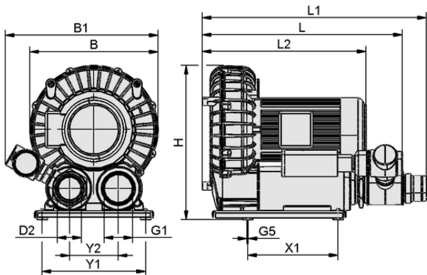
Données de construction SB 375 390 5.5 IE3-TYP1
