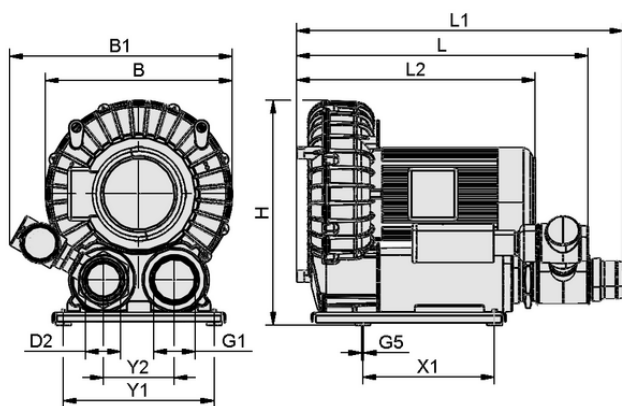
Données de construction SB 1050 290 11 IE3-TYP3
