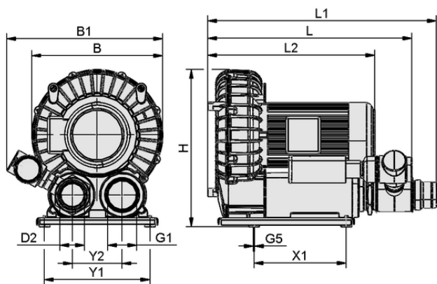
Données de construction SB 1050 290 11 IE3-TYP1
