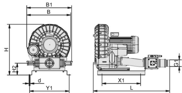
Design data SB 305 400 4.8 IE3-TYP2 ER
