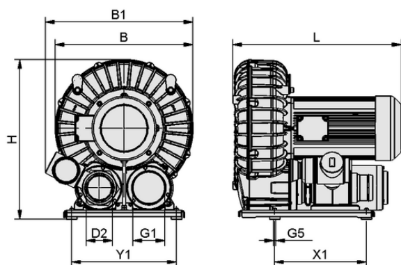
デザインデータ SB 510 390 11 IE3-TYP1
