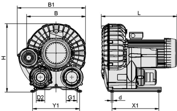
Datos de diseño SB 510 200 4 IE3-TYP1
